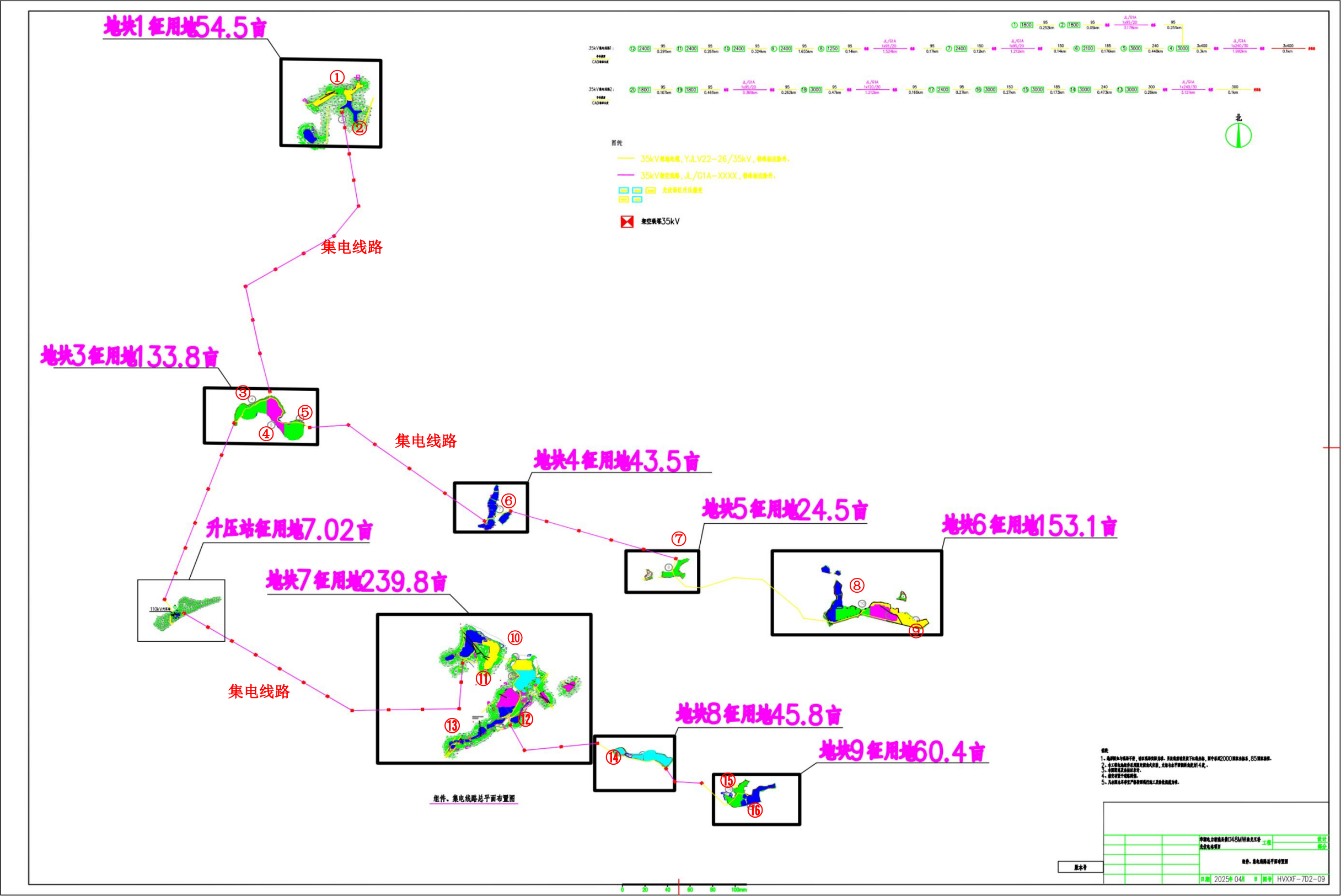
附图四：光伏电站桩位总平布置图
